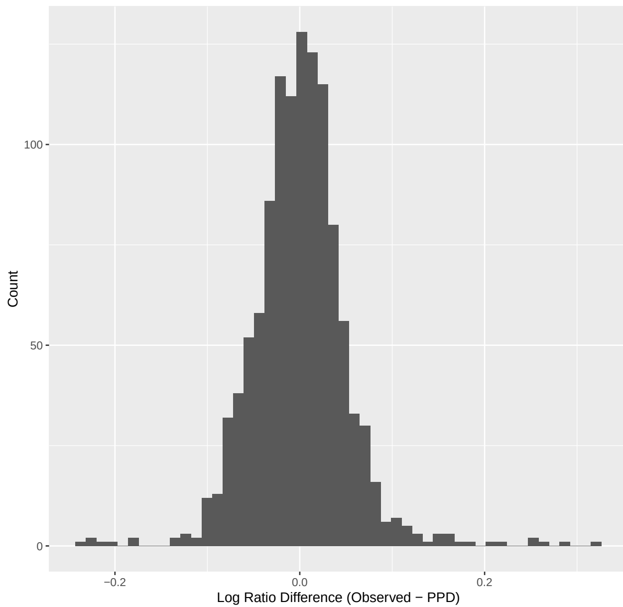
B) Posterior predictive check distribution
